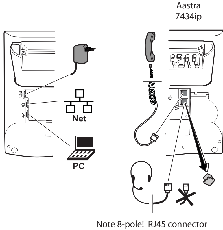
Figure 2: Aastra 7434ip Back View
