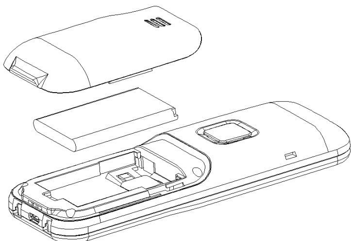
Vložte baterii
